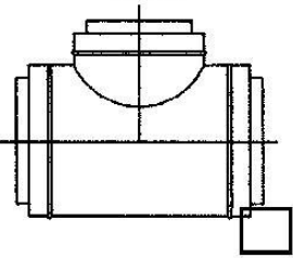
BULLHEAD TEE DW- BH
